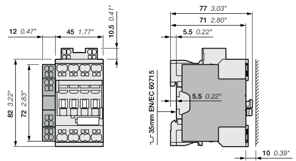
NF22EK, NF31EK, NF40EK + CAL4-11K (2-полюсный контактный блок)
