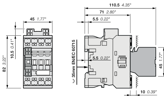
NF22EK, NF31EK, NF40EK + CA4..K (1-полюсный контактный блок)
