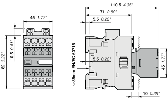
NF22EK, NF31EK, NF40EK + CA4..K (4-полюсный контактный блок)
